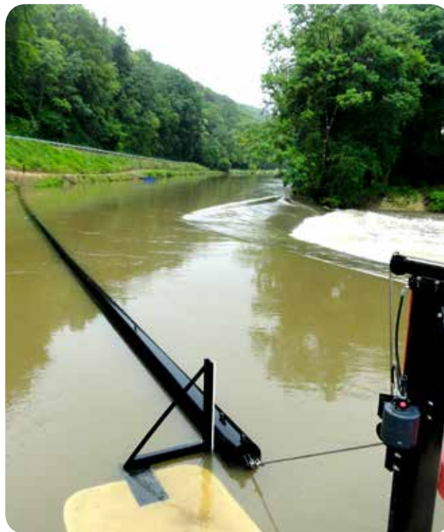
➤ Drome (avec système de contrepoids) pour détourner les objets flottants - Centrale de Ray-sur-Saône (70)
