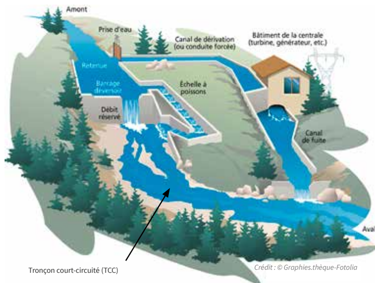
▷ Schéma d'une installation sur canal de dérivation
